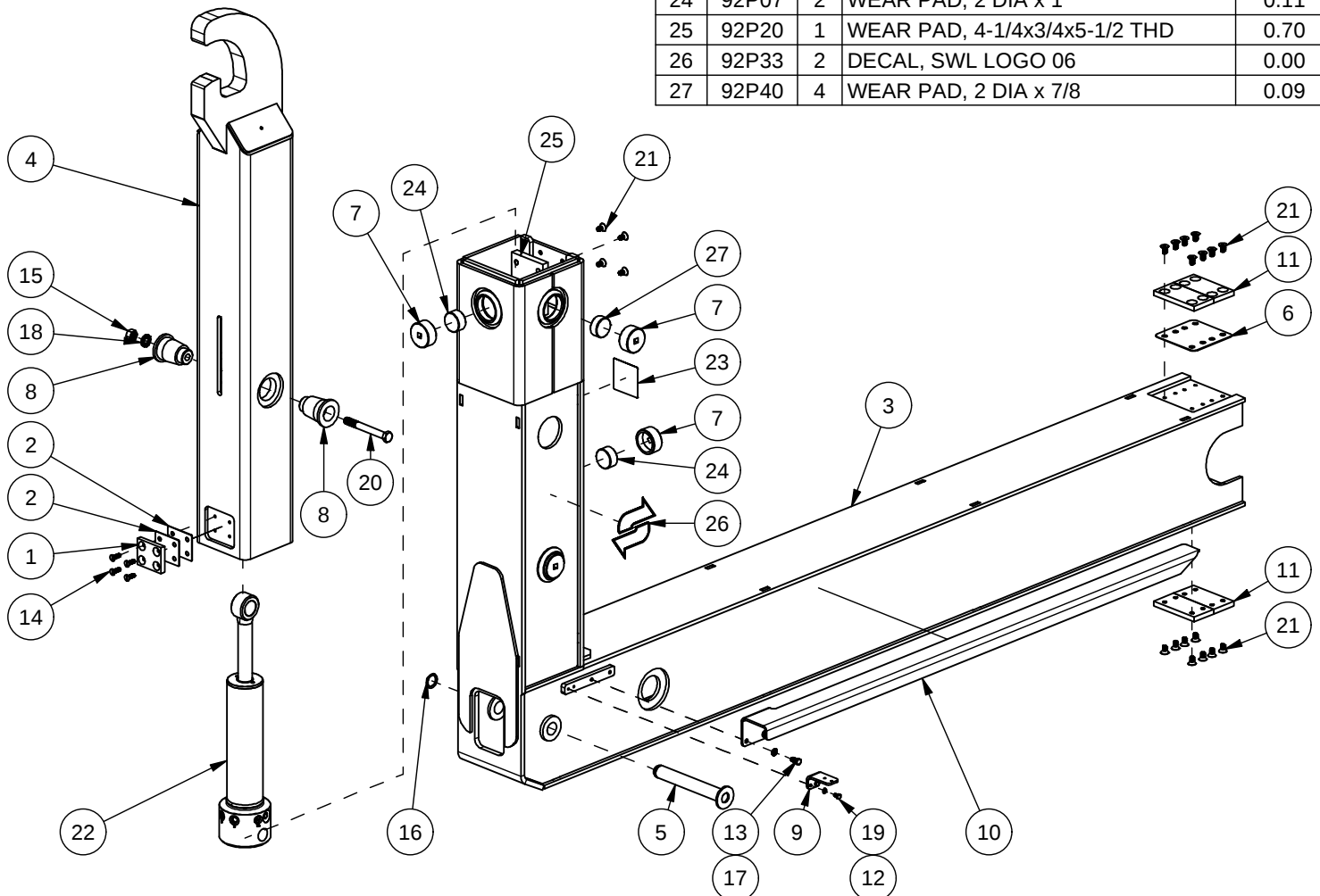
HYD JIB SUB-ASSY, SL-520X
